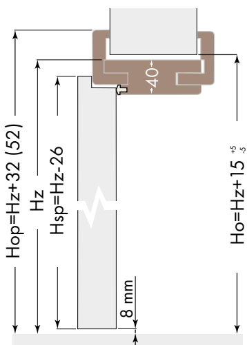
Ościeznica z panelem
