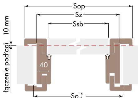
Ościeznica regulowana opaski 60 (80)mm skrzydło bezprzylgowe
