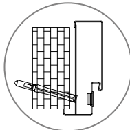
otwór montażowy kotwy w fелcu ościeżnicy
