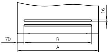
szczelina wentylacyjna w skrzydłach o konstrukcji płytowej – dopłata 70/86,10
