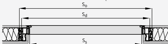
DRZWI OTWIERANE DO WEWNĄTRZ ODW
