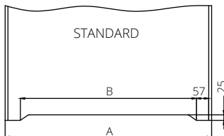
podcięcie wentylacyjne w skrzydłach przylgowych - dopłata powierzchnie fornirowane 50/61,50 - dopłata powierzchnie syntetyczne/malowane 35/43,05
