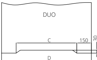
podcięcie wentylacyjne w skrzydłach bezprzylgowych z kolekcji DUO - dopłata powierzchnie fornirowane 50/61,50 - dopłata powierzchnie syntetyczne/malowane 35/43,05
